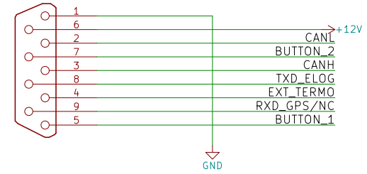
XT1 Дополнительный разъем DB9
