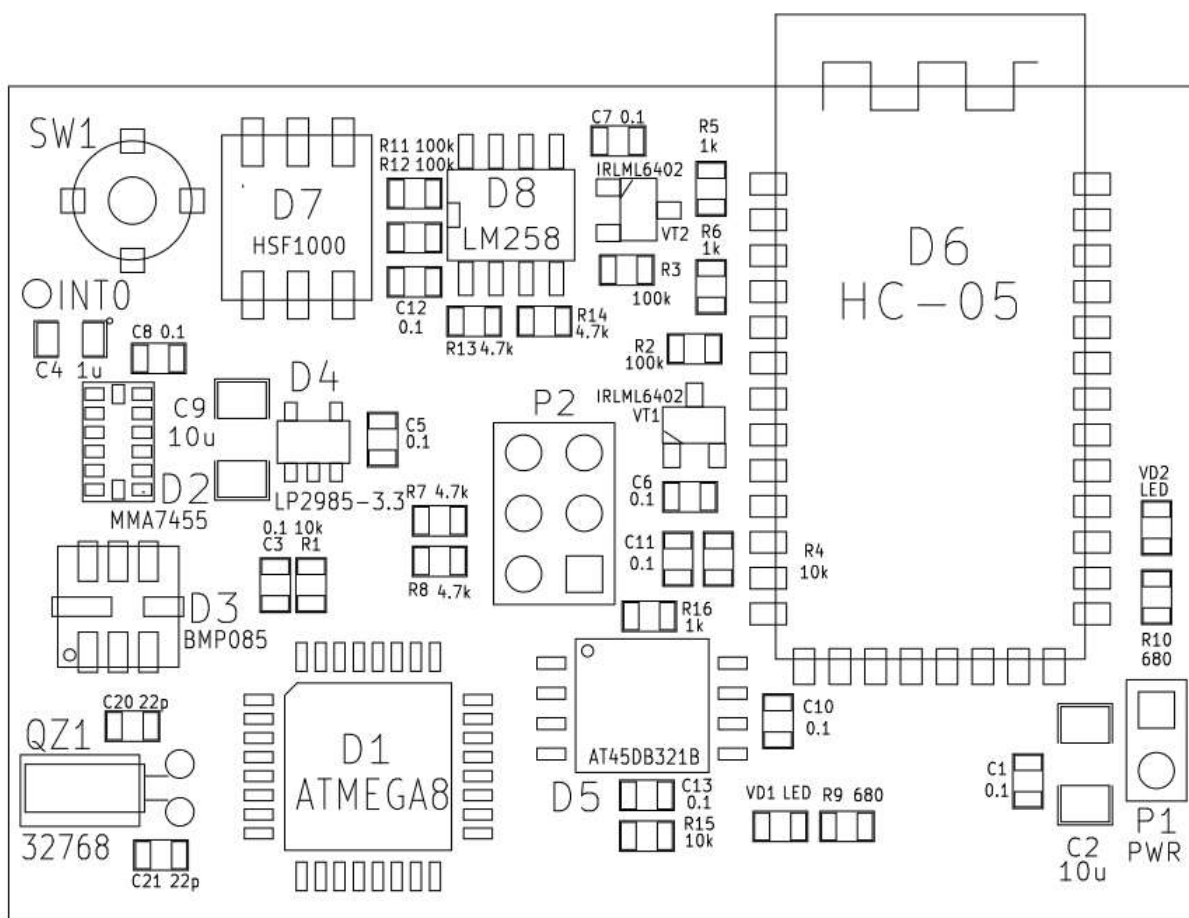
Рисунок 2 - Сборочный чертеж
